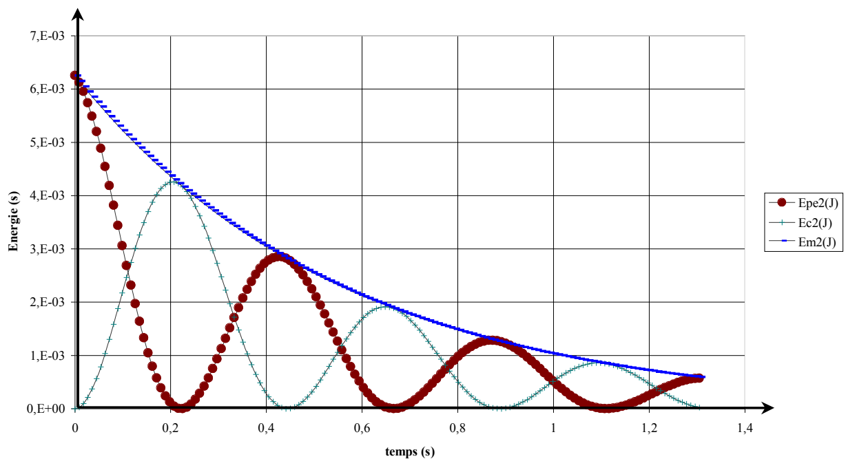
Energie d'un système ressort solide Oscillations avec frottements
