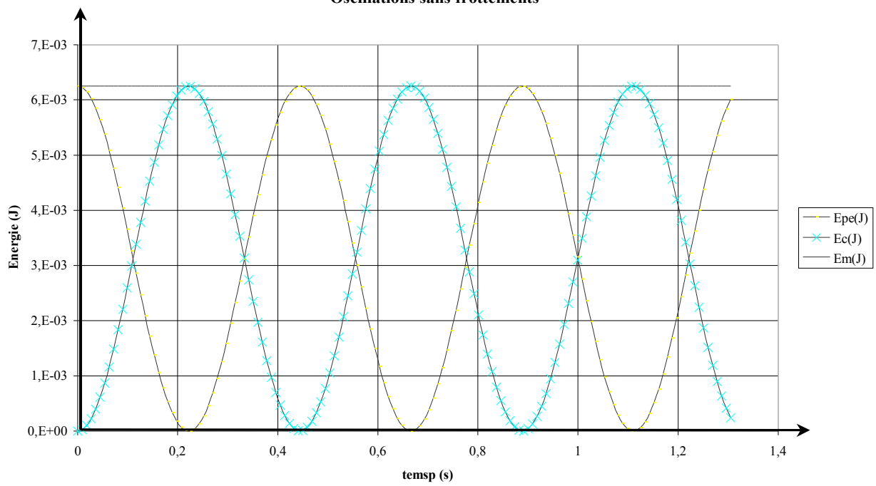
Energie du système ressort Solide Oscillations sans frottements
